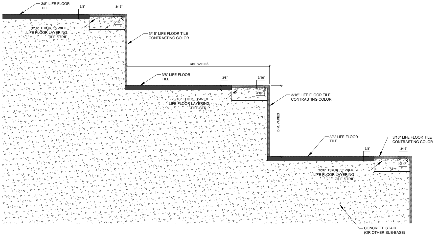
1 LIFE FLOOR STAIR WRAP VARIANT 1 SCALE: 3" = 1'-0"
